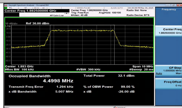
Band25-5MHz-QPSK-26365-25RB#0-PASS
