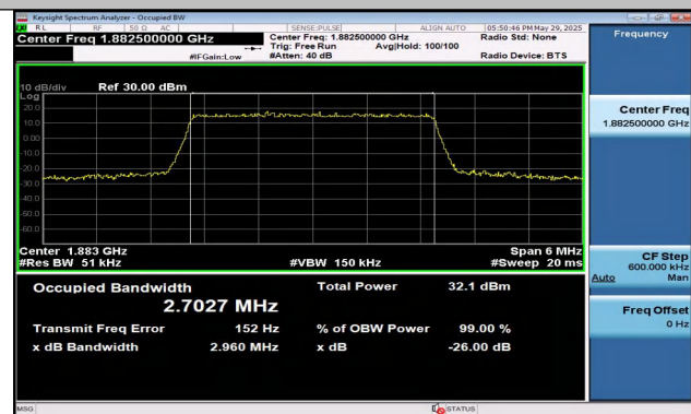
Band25-3MHz-QPSK-26365-15RB#0-PASS
