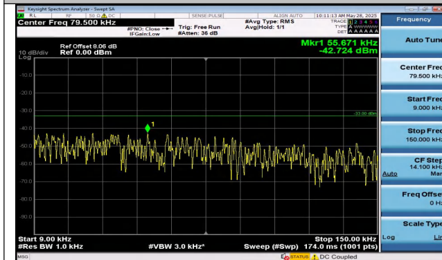
Band5-3MHz-QPSK-20635-1RB#0-0.009~0.15-PASS
