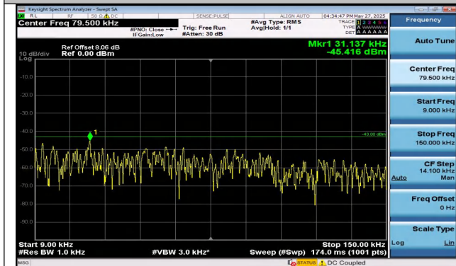
Band4-10MHz-QPSK-20000-50RB#0-0.009~0.15-PASS
