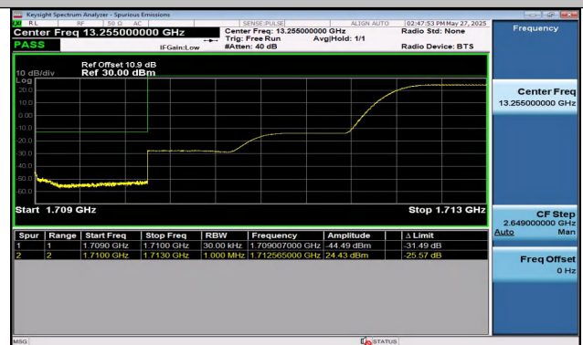
Band4-3MHz-QPSK-19965-1RB#14-PASS
