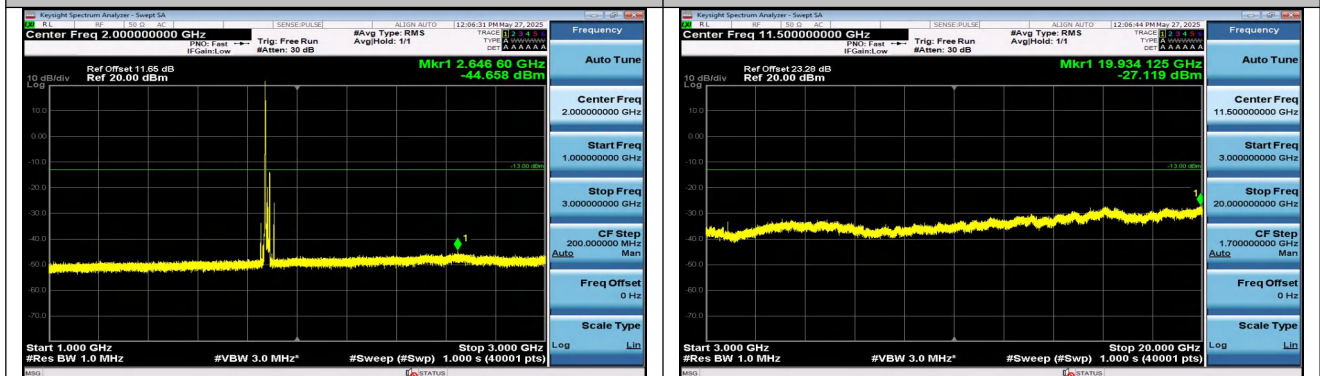
Band2-20MHz-QPSK-18900-1RB#0-1000~3000-PASS
