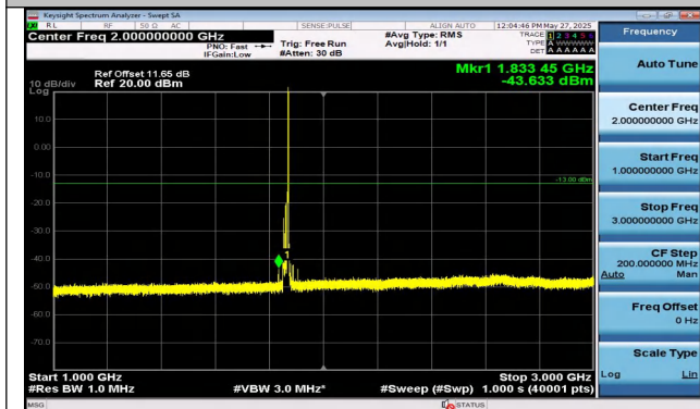
Band2-20MHz-QPSK-18700-1RB#99-1000~3000-PASS
