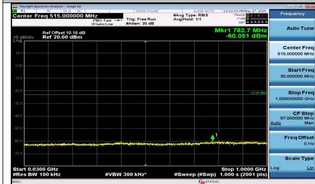
Band2-20MHz-QPSK-18700-1RB#0-30~1000-PASS
