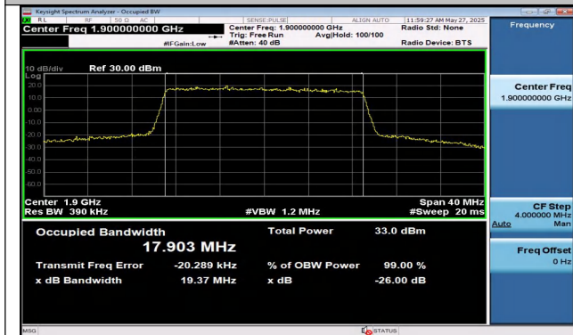
Band2-20MHz-QPSK-19100-100RB#0-PASS
