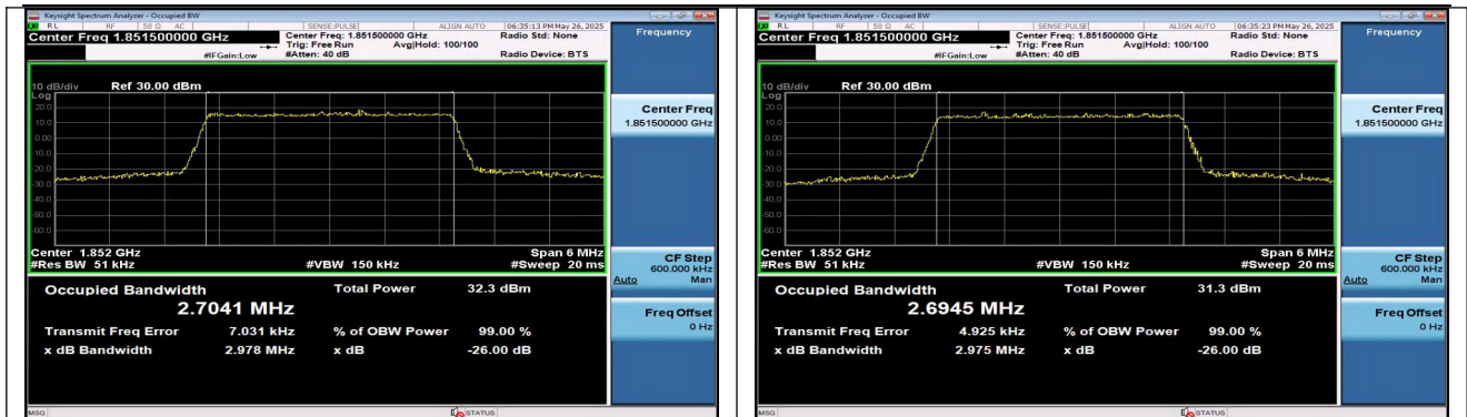
Band2-3MHz-QPSK-18615-15RB#0-PASS
