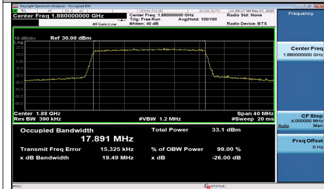
Band2-20MHz-QPSK-18900-100RB#0-PASS
