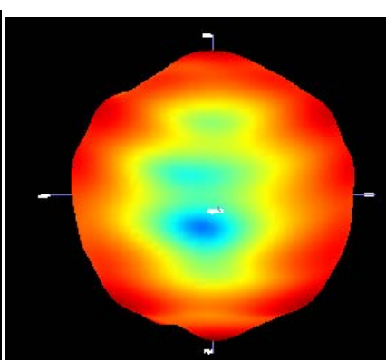
XOZ
