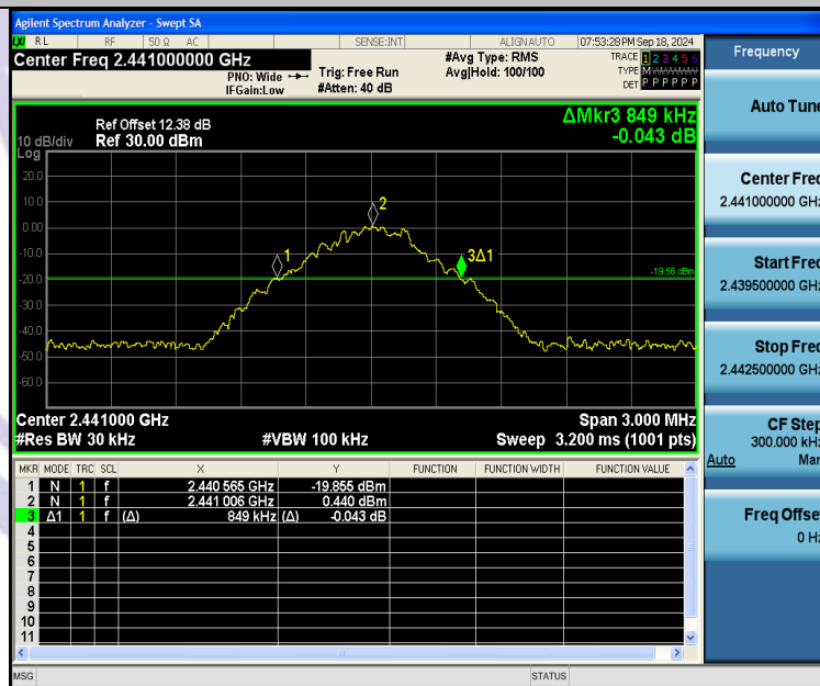
DH5-Ant1-2441
