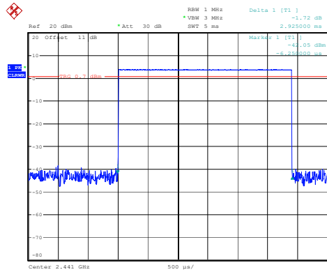
DH5_Hopping 2.925ms
