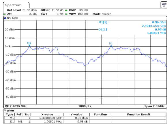
DH1_Hop 1.005MHz
