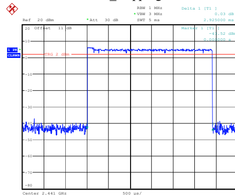
2DH5_Hopping 2.925ms
