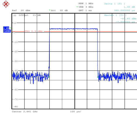
DH1_Hopping 0.395ms
