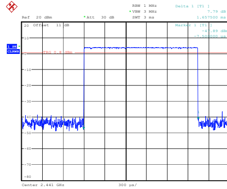
DH3_Hopping 1.658ms
