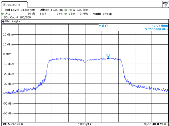
802.11ac20_5745MHz
