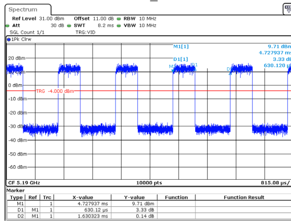
802.11ac40_5190MHz
