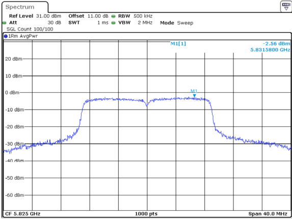
802.11ac20_5825MHz
