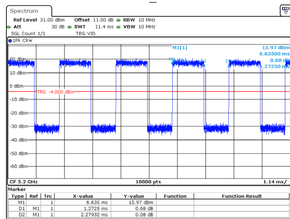
802.11ac20_5200MHz
