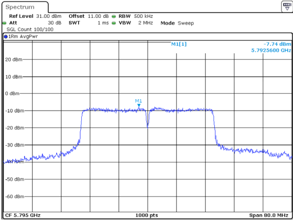
802.11ac40_5795MHz
