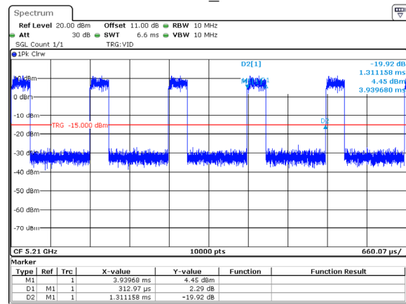
802.11ac80_5210MHz
