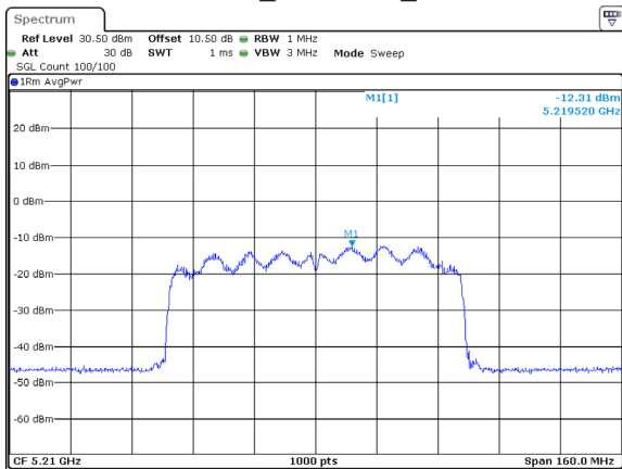
802.11ac80_5210MHz_Chain 0
