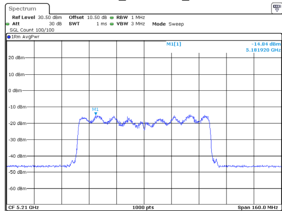
802.11ac80_5210MHz_Chain 1
