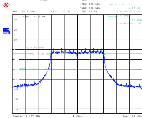
802.11g_2437MHz_Chain 1 16.400MHz
