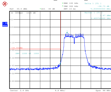
802.11n20_2412MHz_Chain 0
