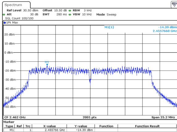
802.11n20_2462MHz_Chain 1 -14.39dBm/3kHz
