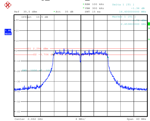
802.11g_2462MHz_Chain 1 16.400MHz
