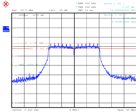
802.11g_2412MHz_Chain 0 16.400MHz
