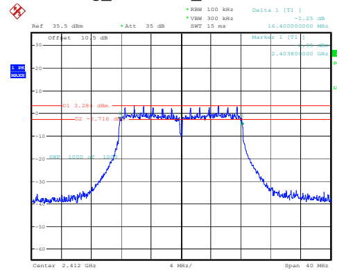
802.11g_2412MHz_Chain 1 16.400MHz
