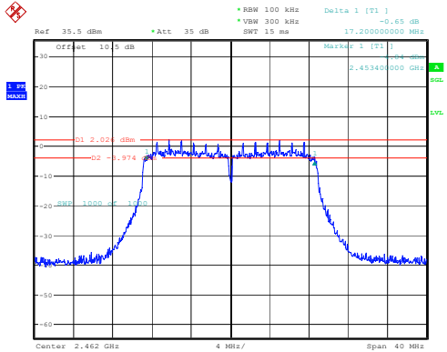
802.11n20_2462MHz_Chain 0 17.200MHz
