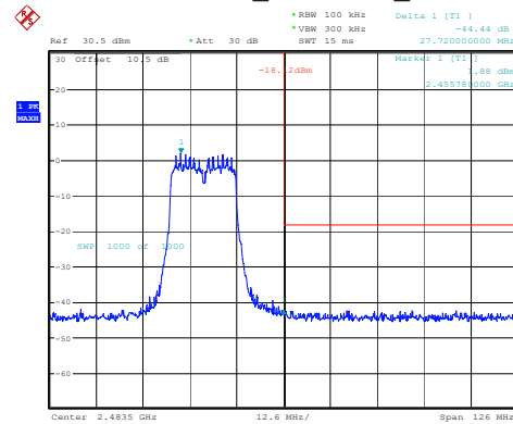
802.11n20_2462MHz_Chain 0
