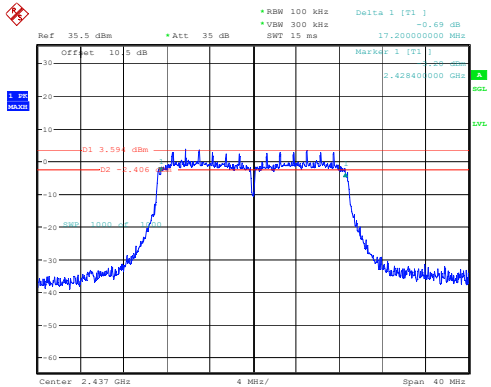
802.11n20_2437MHz_Chain 0 17.200MHz
