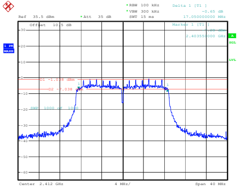
802.11n20_2412MHz_Chain 1 17.050MHz
