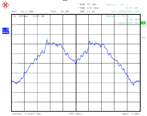
DH1_Low 0.998MHz
