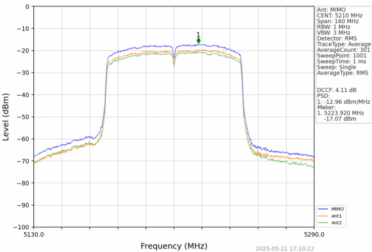
802.11ac(VHT80)_MCH_5210MHz_MIMO_NTNV
