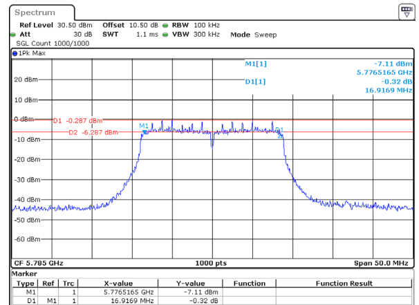
802.11ac20_5785MHz_Chain 0
