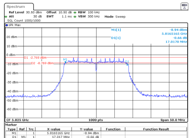
802.11ac20_5825MHz_Chain 1
