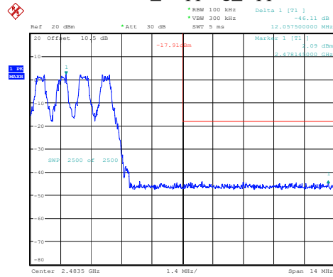
DH1_Hopping_Upper
