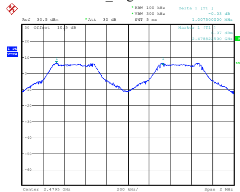
DH1_High 1.008MHz
