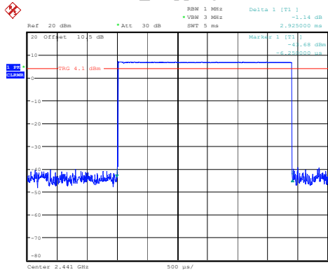
DH5_Hopping 2.925ms
