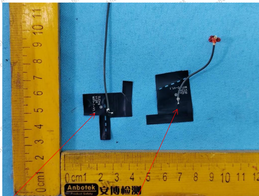
BT/WiFi ANT 1
