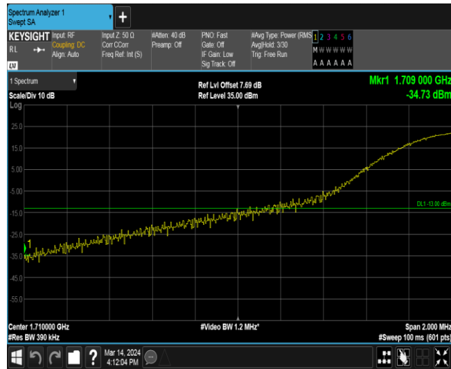
Band66-20MHz-QPSK-132072-1RB#99
