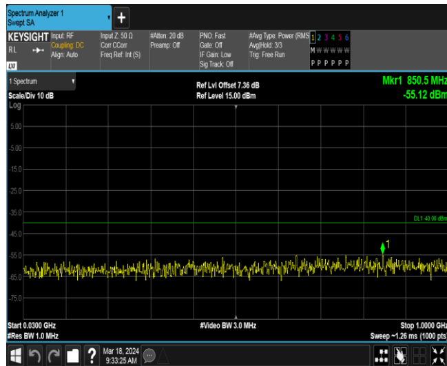
Band40-5MHz-16QAM-38750-1RB#0-Range2:1000~2288MHz
