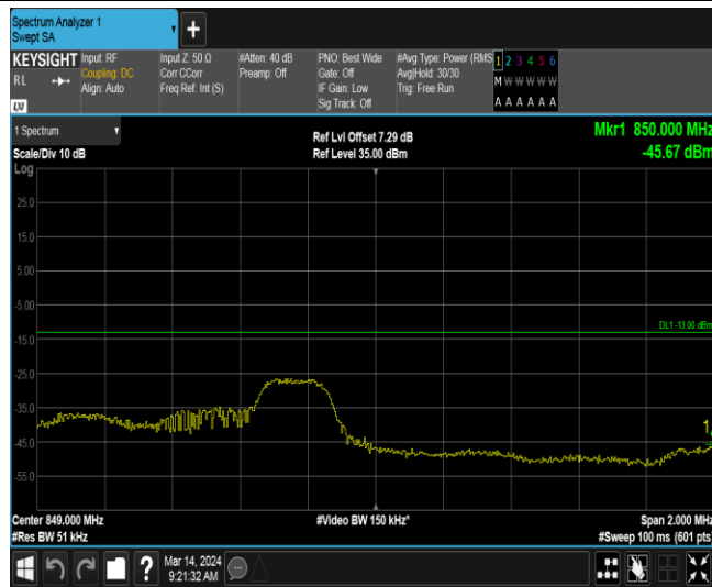
Band5-3MHz-QPSK-20635-1RB#14
