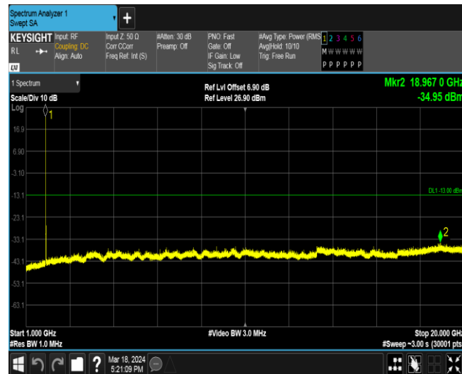
Band2-9400-1-1000~20000MHz
