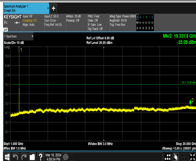
Band2-9538-1-1000~20000MHz
