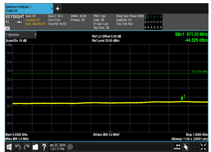
EGPRS1900-810-2-30~1000MHz-PASS
