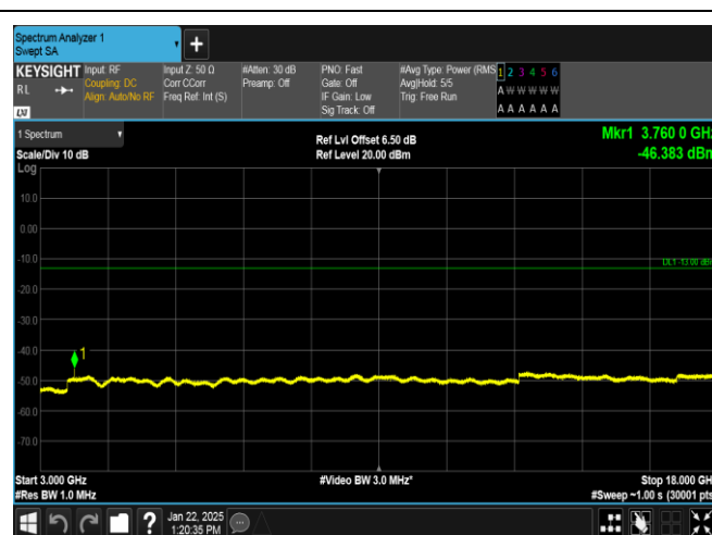
EGPRS1900-661-2-3000~18000MHz-PASS
