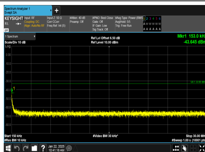
GPRS1900-810-0-0.15~30MHz-PASS
