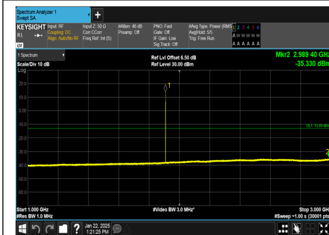
EGPRS1900-810-2-1000~3000MHz-PASS
