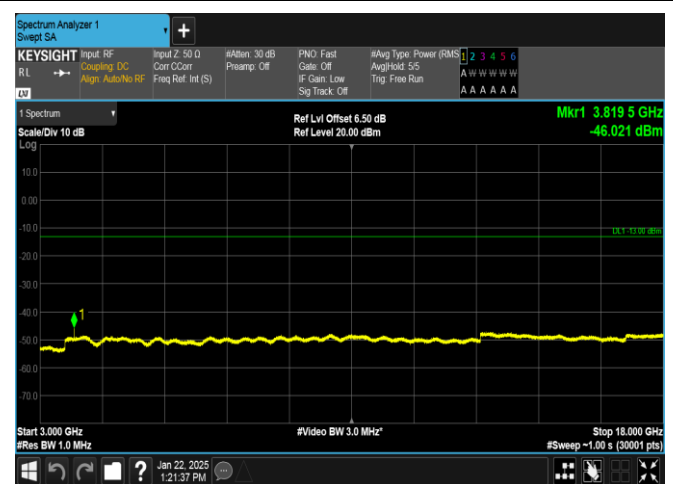
EGPRS1900-810-2-3000~18000MHz-PASS
