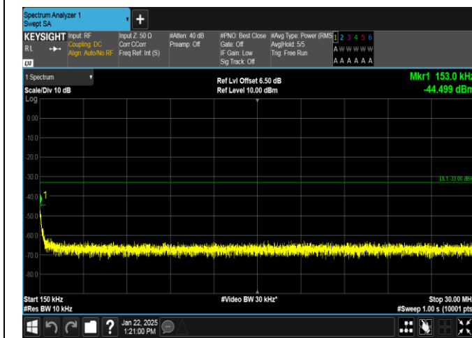
EGPRS1900-810-2-0.15~30MHz-PASS
