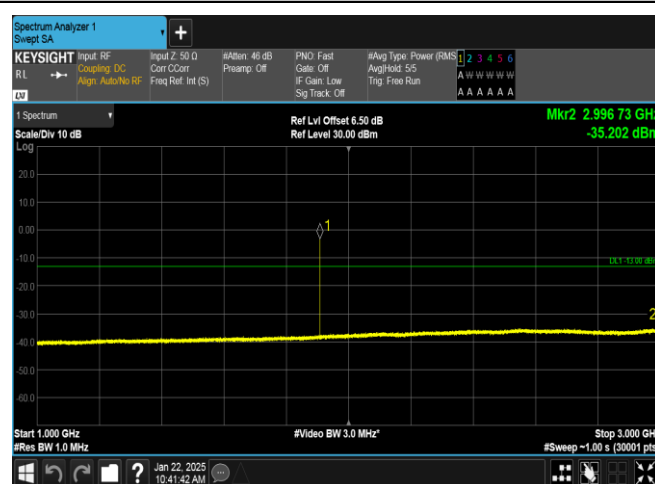
GPRS1900-810-0-1000~3000MHz-PASS
