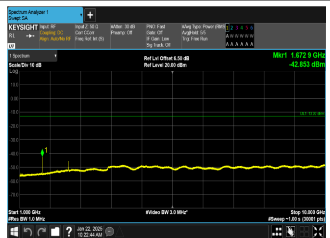
GPRS850-190-5-1000~10000MHz-PASS
