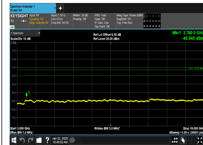
GPRS1900-661-0-3000~18000MHz-PASS
