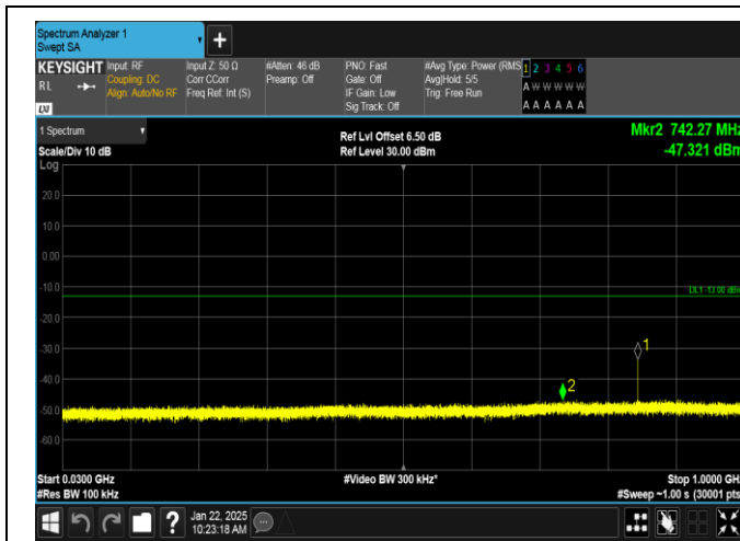
GPRS850-251-5-30~1000MHz-PASS
