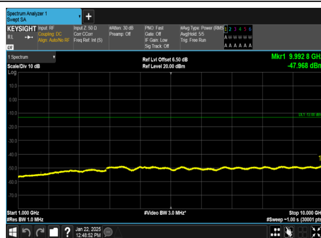
EGPRS850-190-8-1000~10000MHz-PASS
