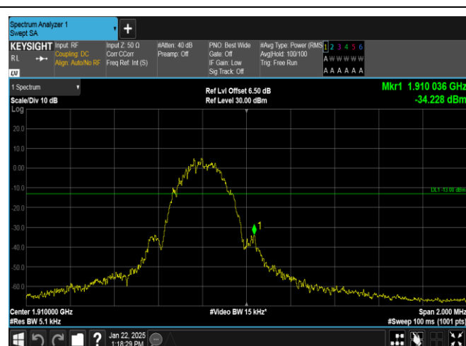
EGPRS1900-810-2-PASS
