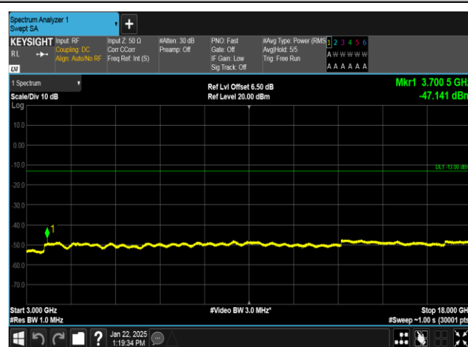
EGPRS1900-512-2-3000~18000MHz-PASS
