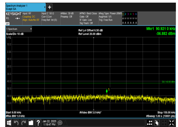
EGPRS1900-661-2-0.009~0.15MHz-PASS
