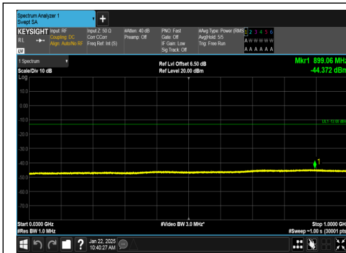
GPRS1900-661-0-30~1000MHz-PASS
