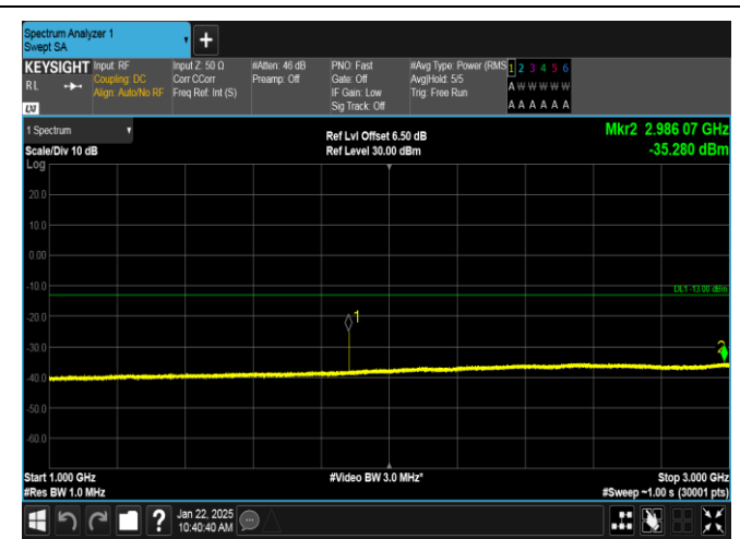
GPRS1900-661-0-1000~3000MHz-PASS
