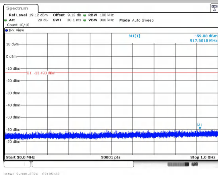
11B_Ant1_2462_30~1000
