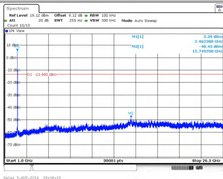
11B_Ant1_2462_1000~26500
