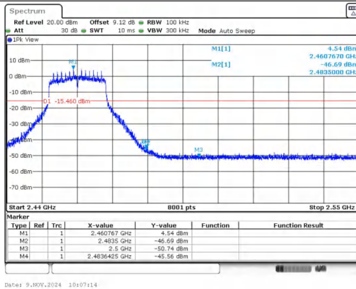
11N20MIMO_Ant1_High_2462
