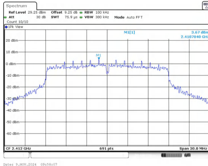
11N20MIMO_Ant2_2412_0~Reference
