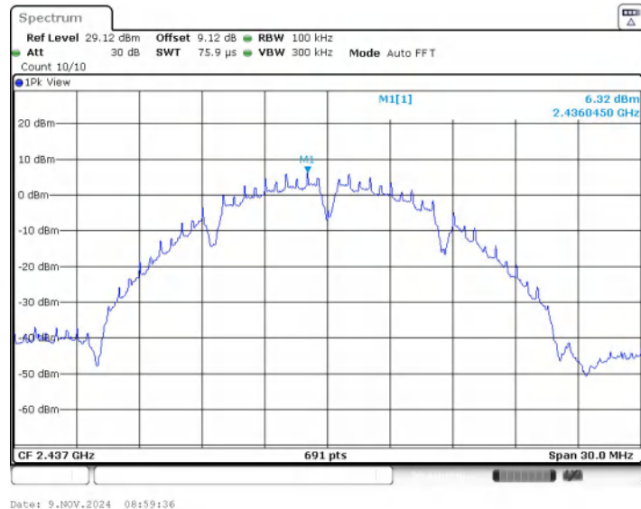
11B_Ant1_2437_0~Reference
