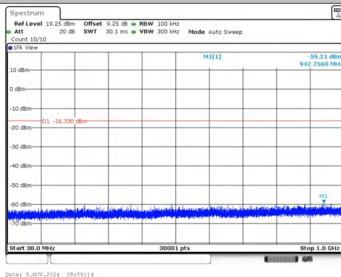
11N20MIMO_Ant2_2412_30~1000
