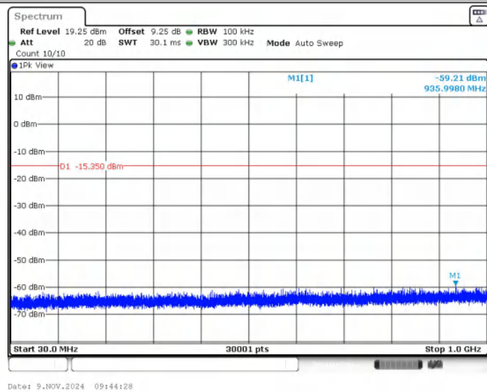
11G_Ant2_2437_30~1000
