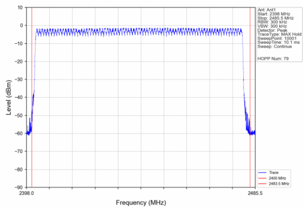
8DPSK
