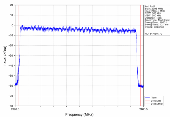
\pi/4 DQPSK
