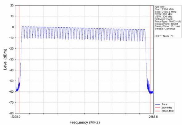
8DPSK
