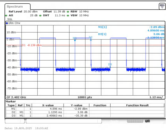
BLE 2M_Channel 0
