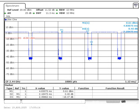
BLE 1M_Channel 19
