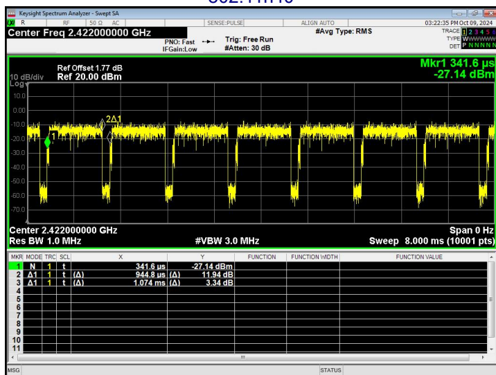
802.11n40
