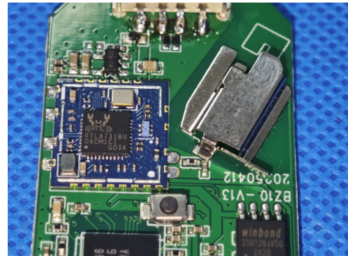
Antenna
