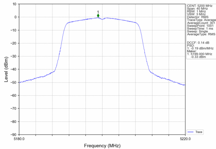
802.11ac(VHT20) MCH 5200MHz_Ant1_NTNV
