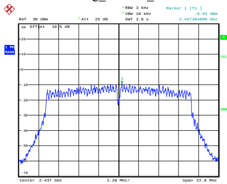
802.11g_Chain 0_2437MHz
