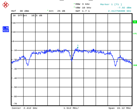
802.11b_Chain 0_2412MHz
