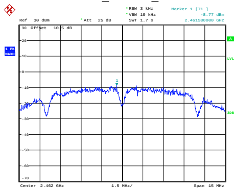
802.11b_Chain 0_2462MHz
