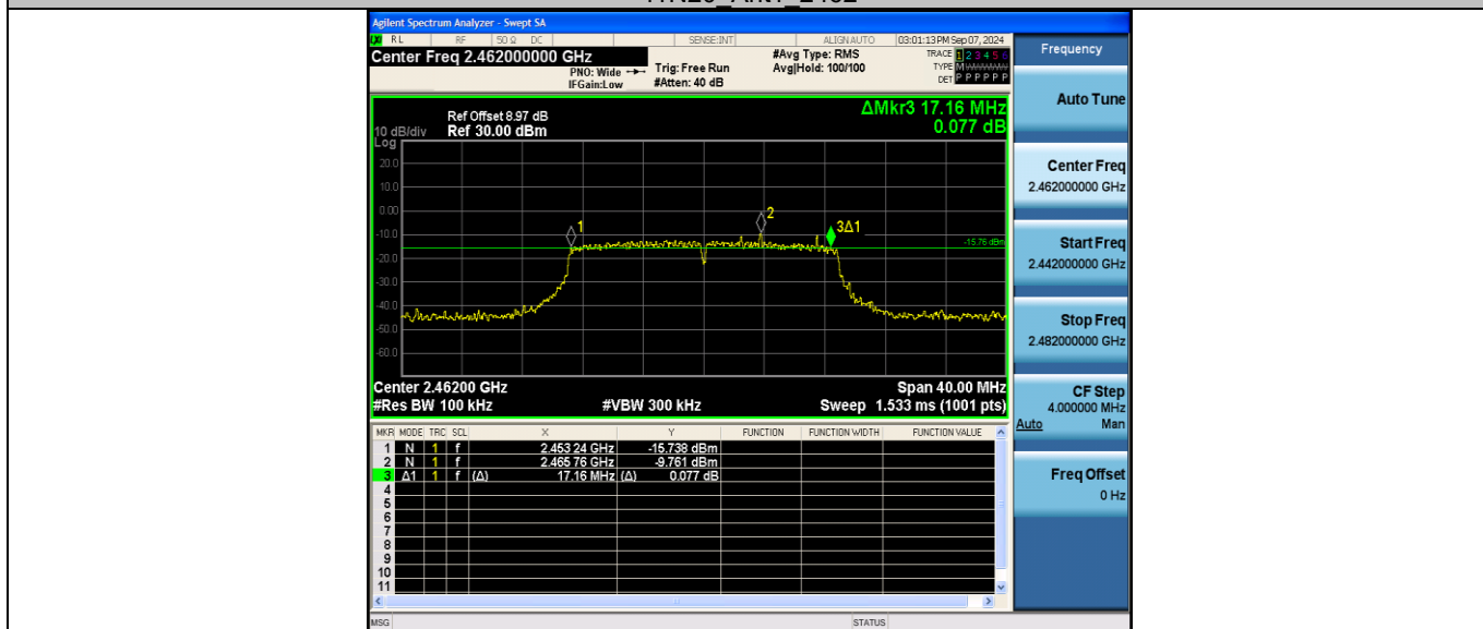
11N20_Ant2_2462
