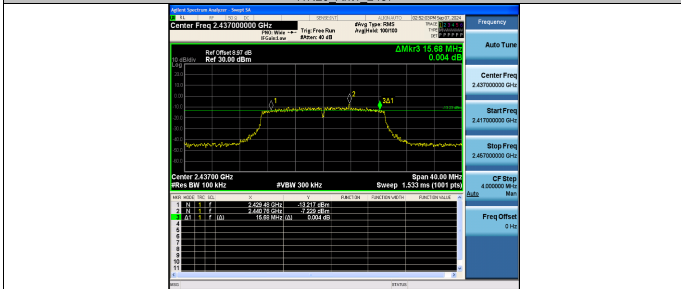
11N20_Ant2_2437
