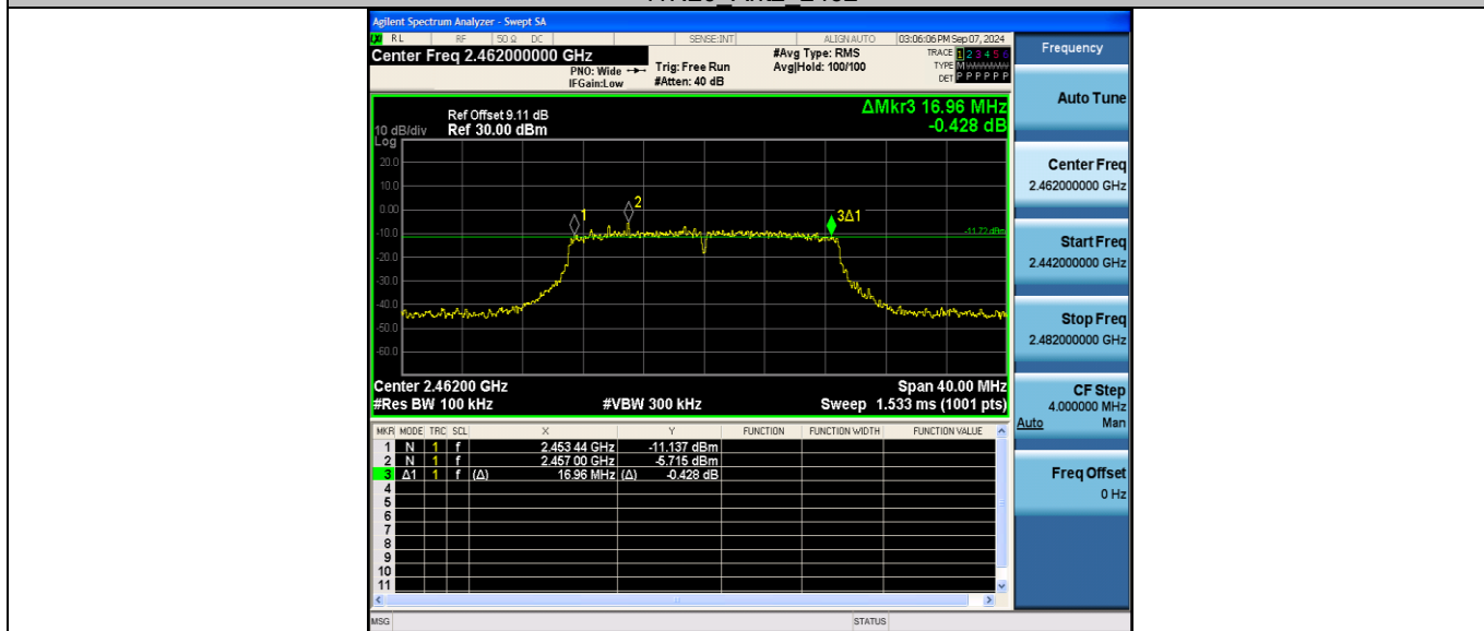
11N20_Ant2_2462
