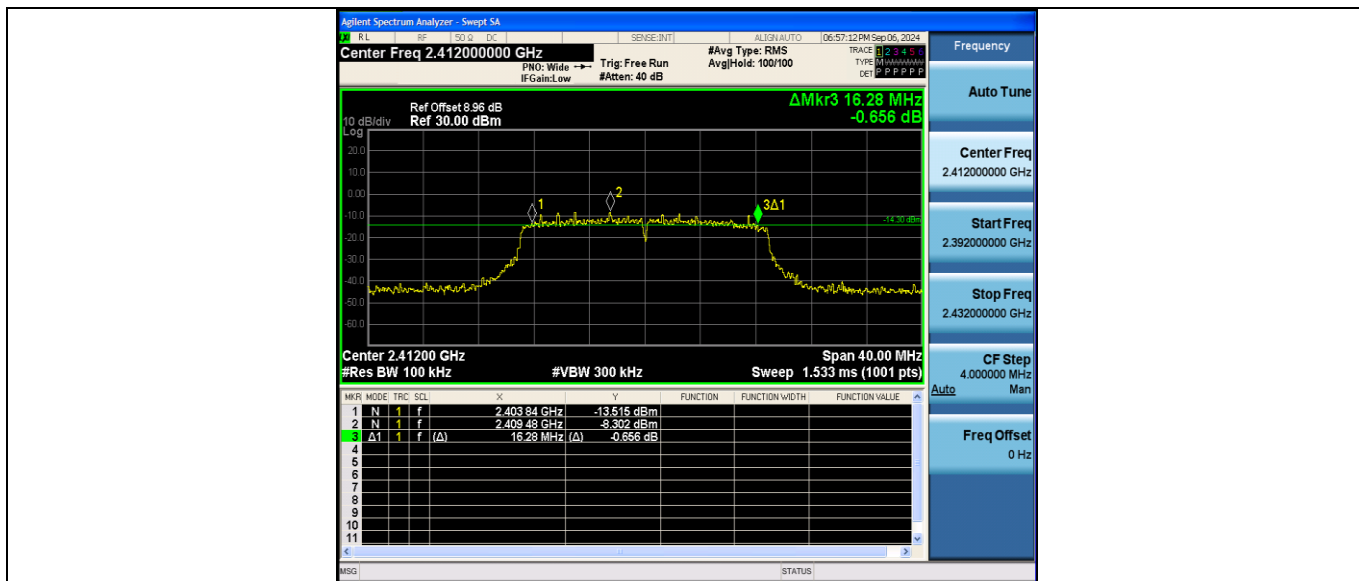
11N20_Ant2_2412
