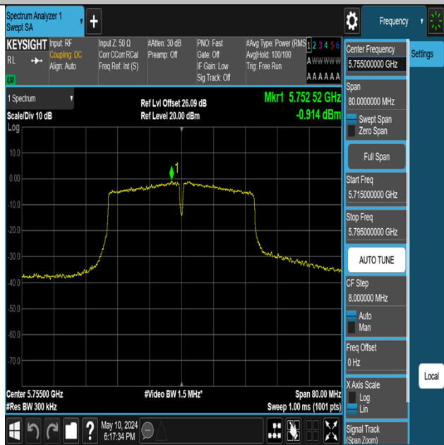
11N40MIMO-Ant1-5755-PASS
