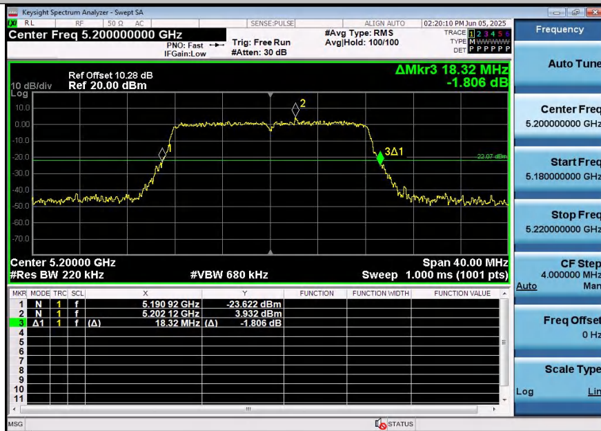
11A-Ant1-5200
