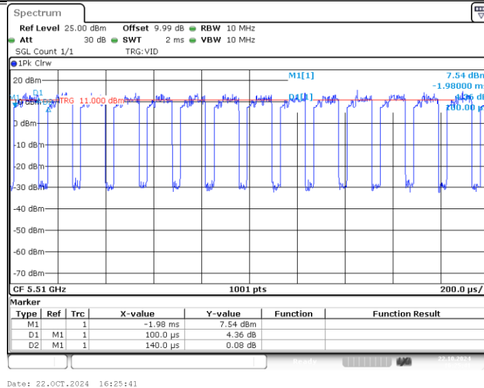
11AX40MIMO_Ant2_5510
