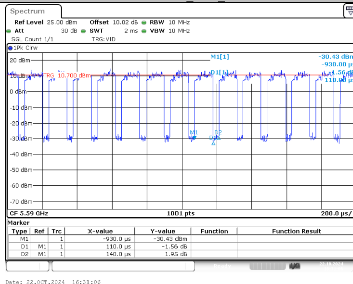
11AX40MIMO_Ant2_5590
