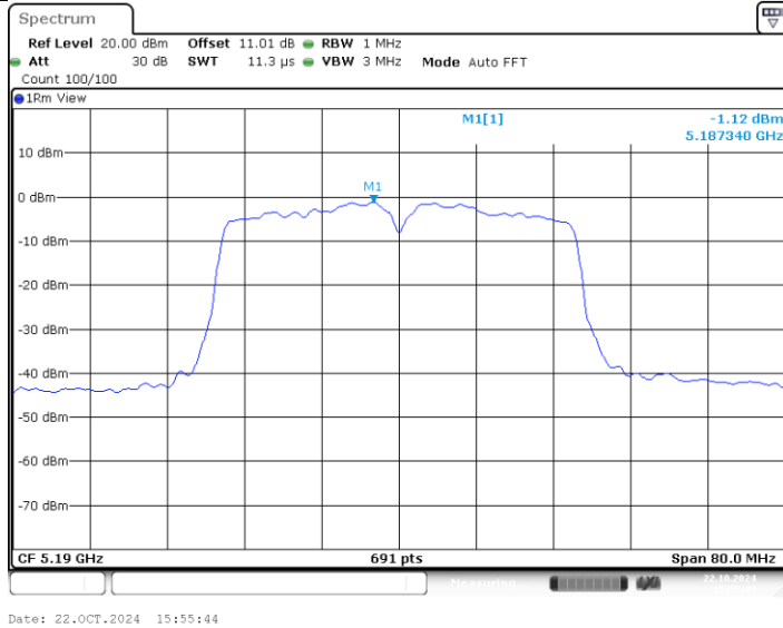
11AX40MIMO_Ant2_5190
