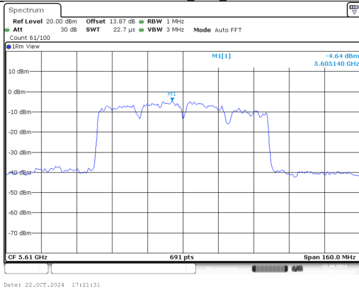
11AX80MIMO_Ant2_5610
