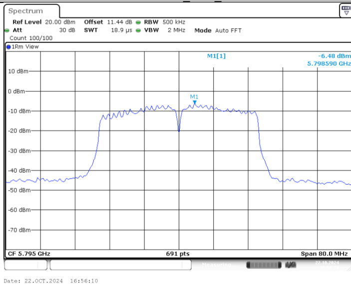
11AX40MIMO_Ant2_5795
