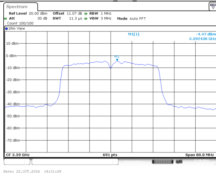
11AX40MIMO_Ant2_5590
