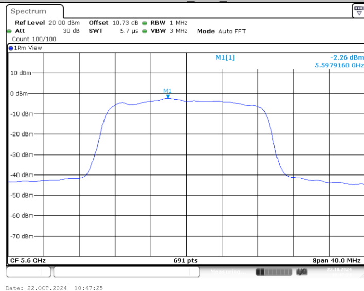
11N20MIMO_Ant2_5600
