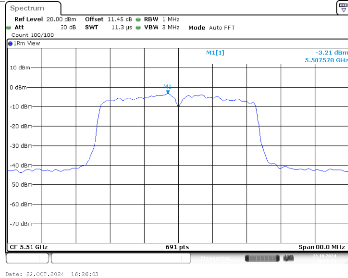
11AX40MIMO_Ant2_5510
