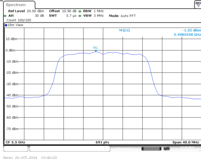
11N20MIMO_Ant2_5500
