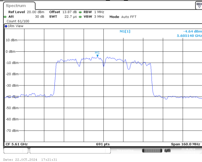
11AX80MIMO_Ant2_5610
