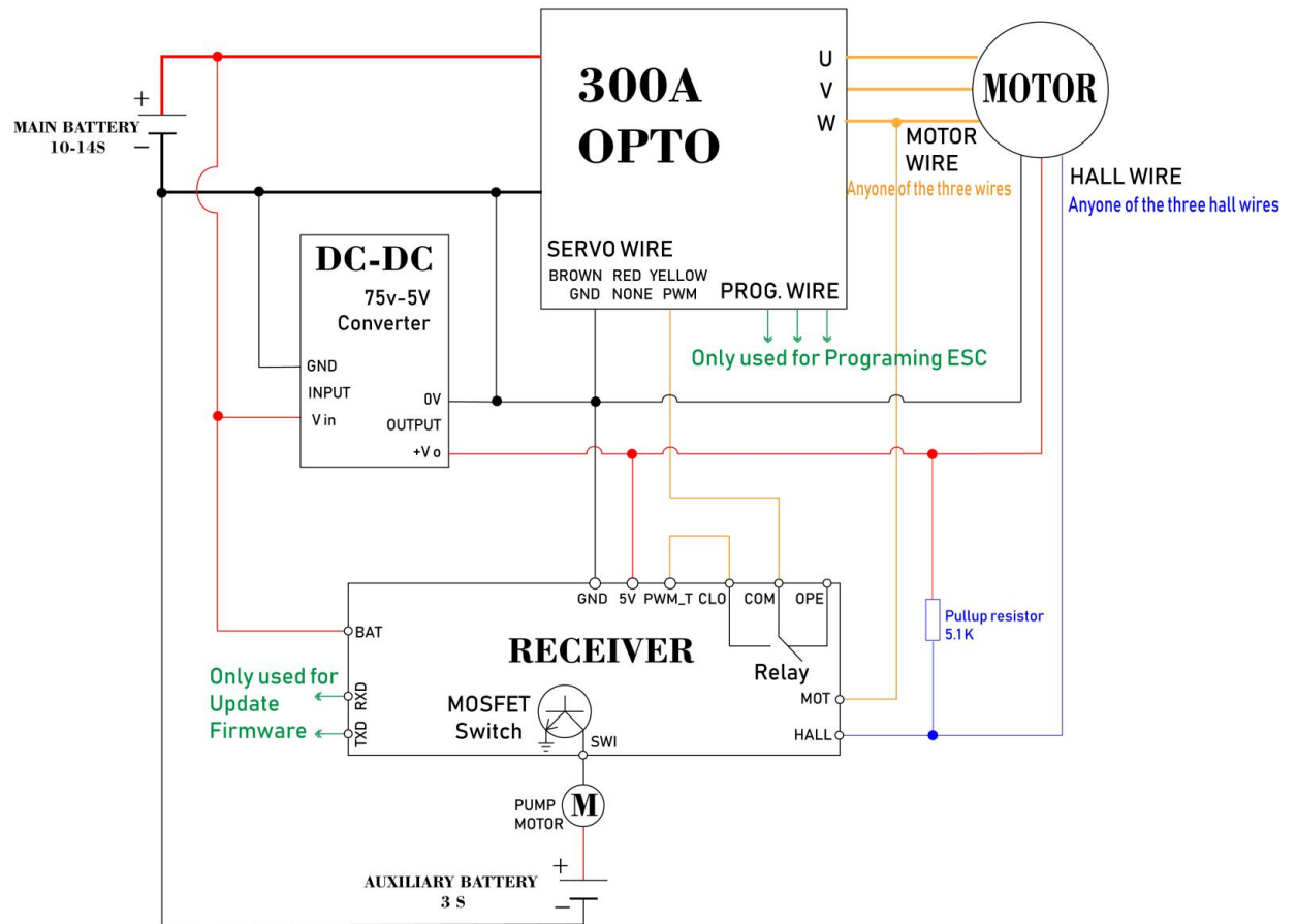
冲浪板电调与接收机全功能连接图，继电器做安全开关
