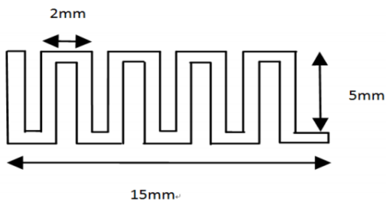
2.4G Ant.
