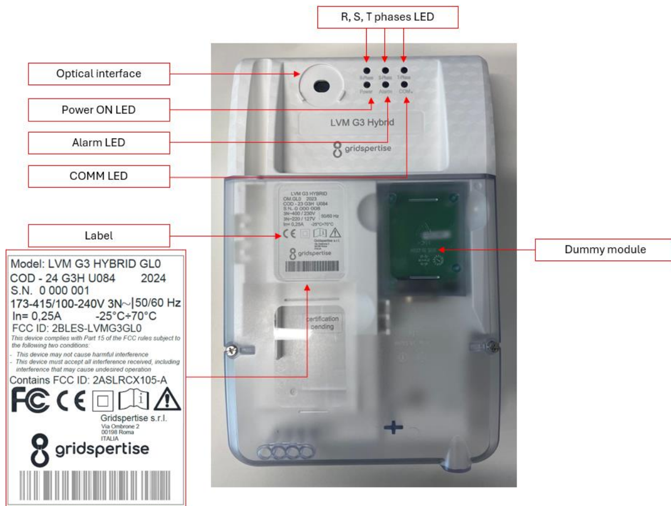
Figura 1 LVM G3 Hybrid GL0
