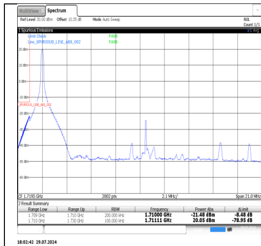
Band66-20MHz-QPSK-132072-1RB#99-PASS
