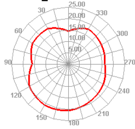
WCDMA_II 9538 TRP Phi=45
