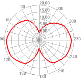
LTE71 133422 TRP Phi=45
