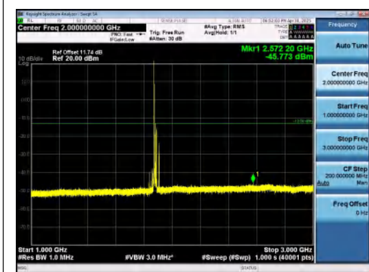
Band2-20MHz-16QAM-18900-1RB#0-1000~300 0-PASS
