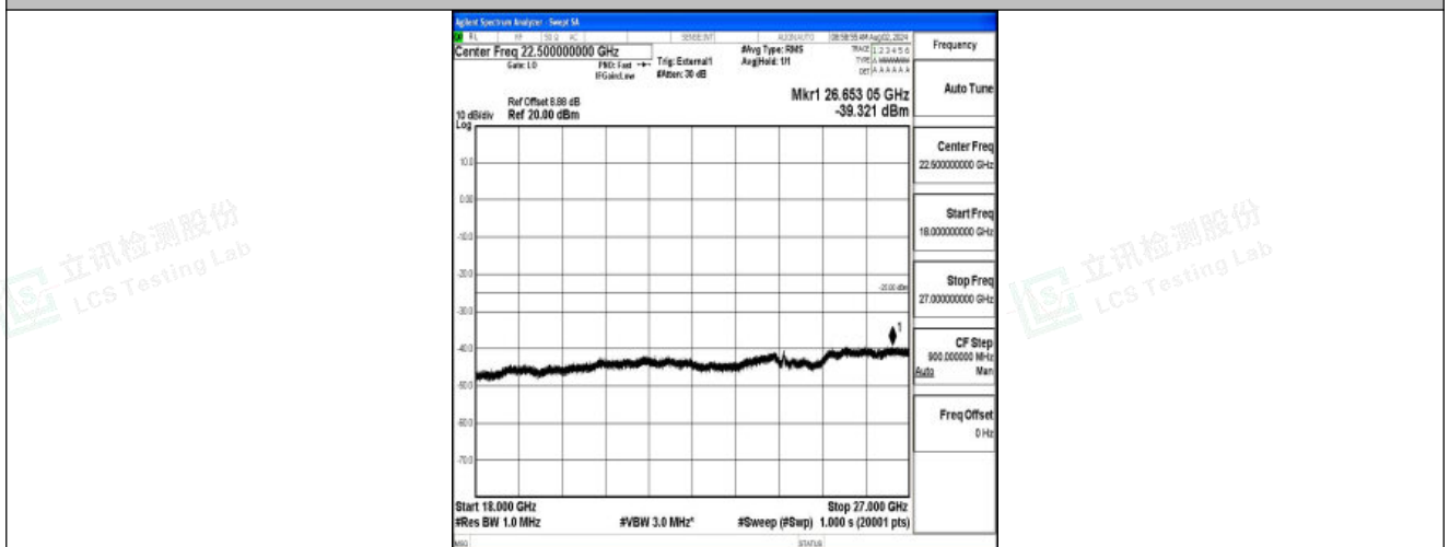
Band41-20MHz-16QAM-41490-1RB#0-18000~27000-PASS
