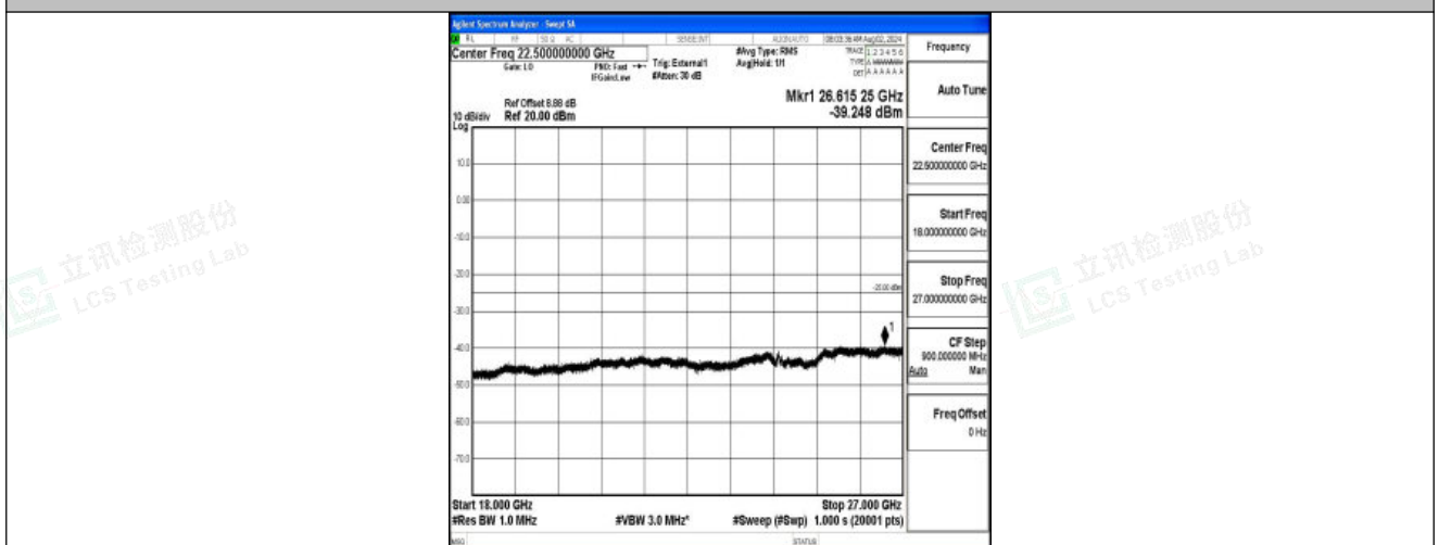
Band41-15MHz-16QAM-39725-1RB#0-18000~27000-PASS
