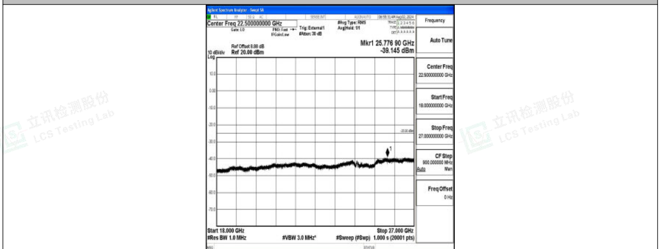
Band41-5MHz-16QAM-41565-1RB#0-18000~27000-PASS
