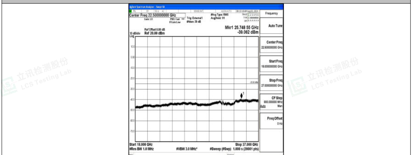
Band41-15MHz-16QAM-41515-1RB#0-18000~27000-PASS
