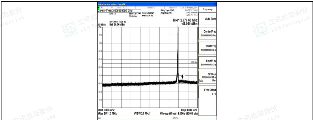
Band38-20MHz-QPSK-37850-1RB#0-1000~3000-PASS
