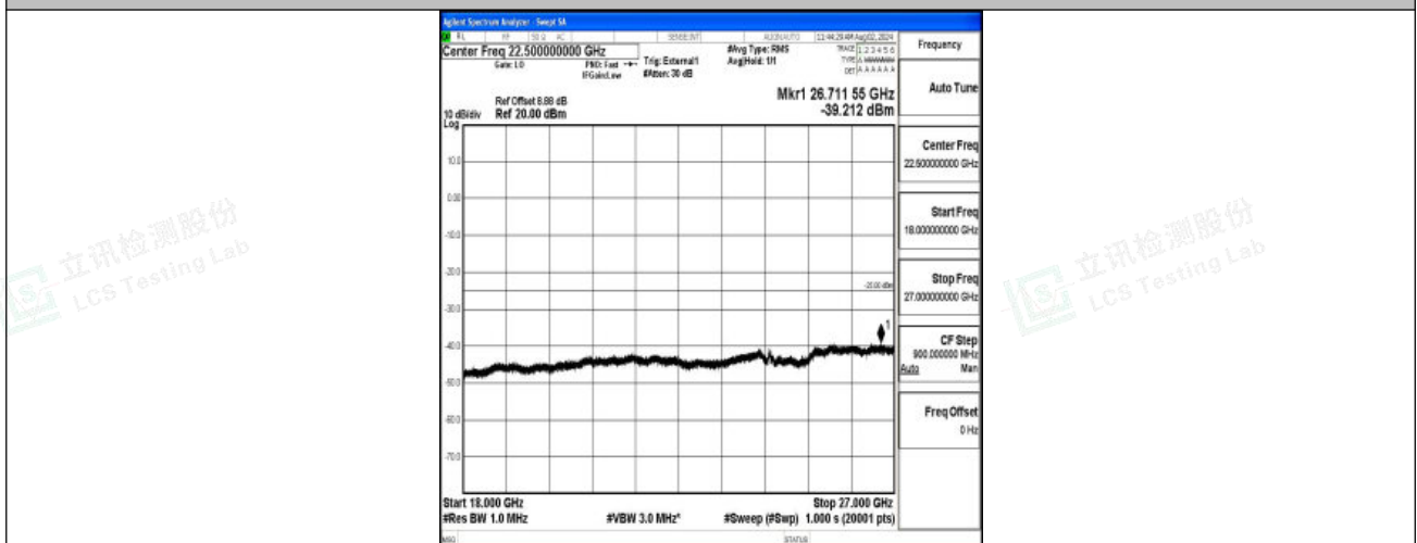
Band38-20MHz-QPSK-37850-1RB#0-18000~27000-PASS
