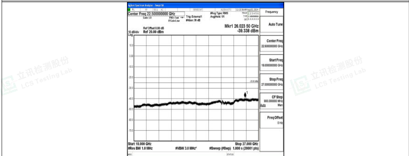
Band38-15MHz-QPSK-37825-1RB#0-18000~27000-PASS
