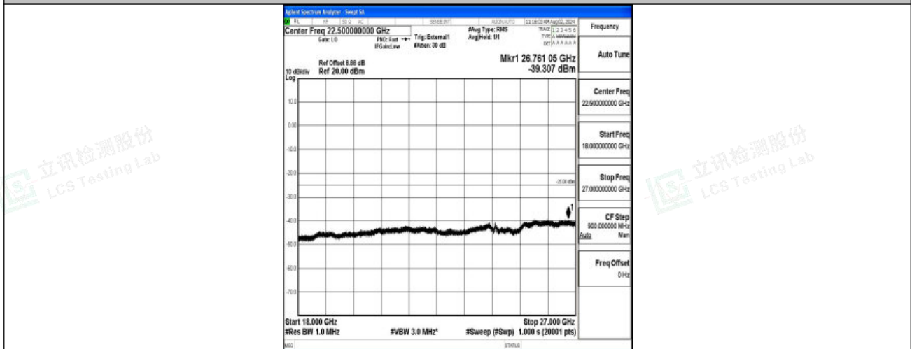
Band38-15MHz-16QAM-37825-1RB#0-18000~27000-PASS
