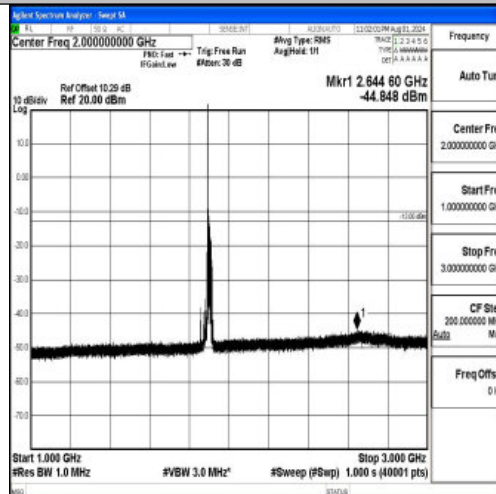
Band2-20MHz-QPSK-19100-1RB#0-1000~3000-PASS
