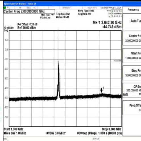
Band2-20MHz-QPSK-18900-1RB#0-1000~3000-PASS
