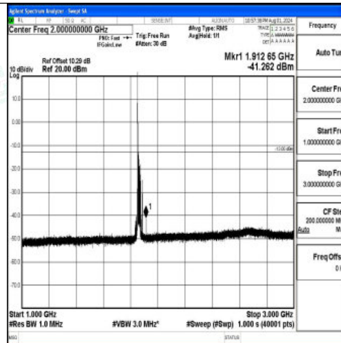
Band2-20MHz-QPSK-18700-1RB#0-1000~3000-PASS
