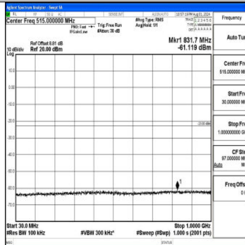
Band2-20MHz-QPSK-18700-1RB#0-30~1000-PASS
