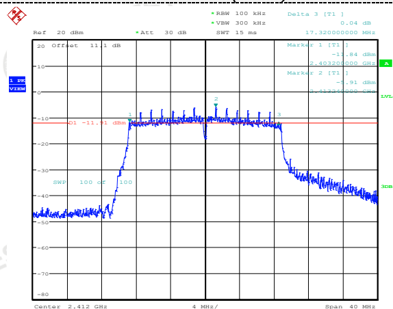
802.11n(HT20)
