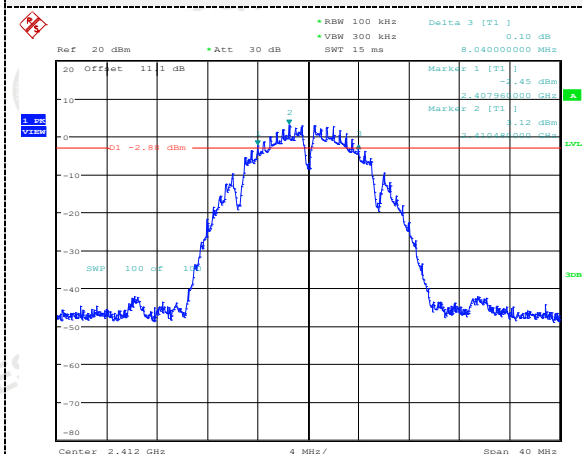
802.11b
