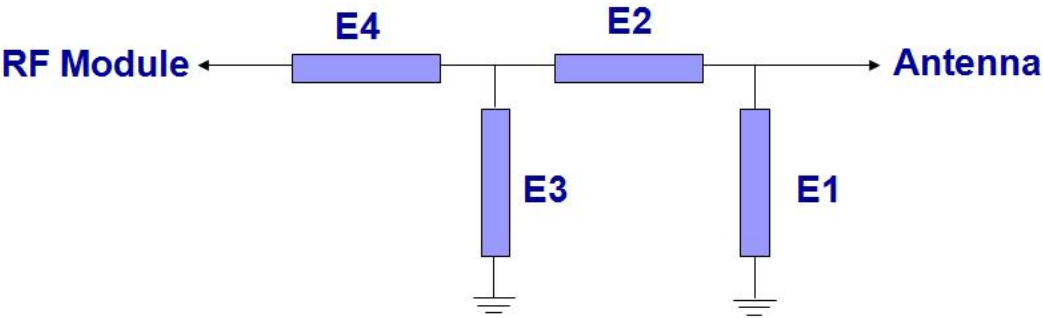
匹配电路
