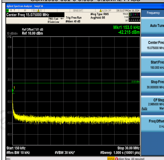
GSM1900-661-0-0.15~30MHz-PASS
