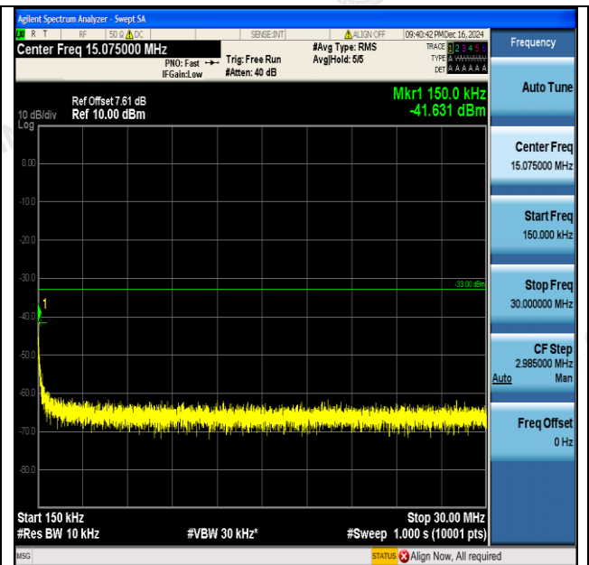
GPRS1900-512-0-0.15-30MHz-PASS
