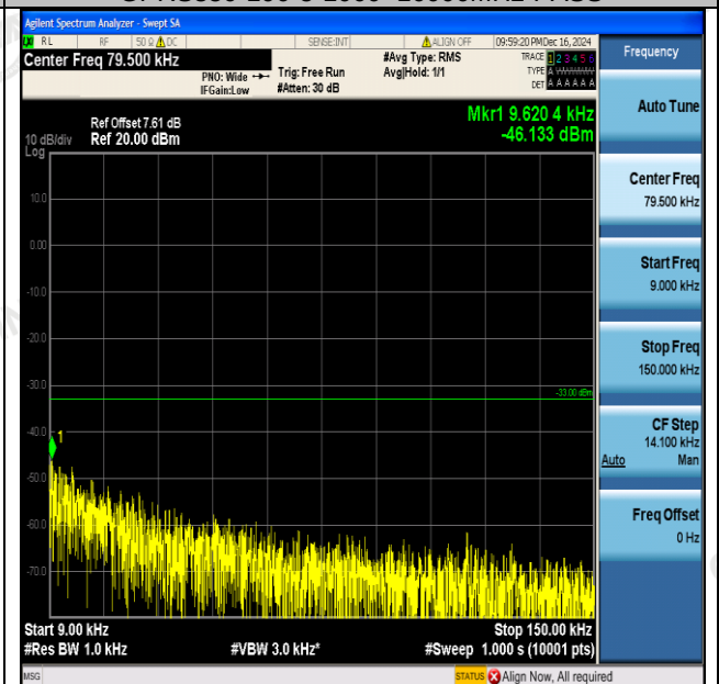
GPRS850-251-5-0.009~0.15MHz-PASS
