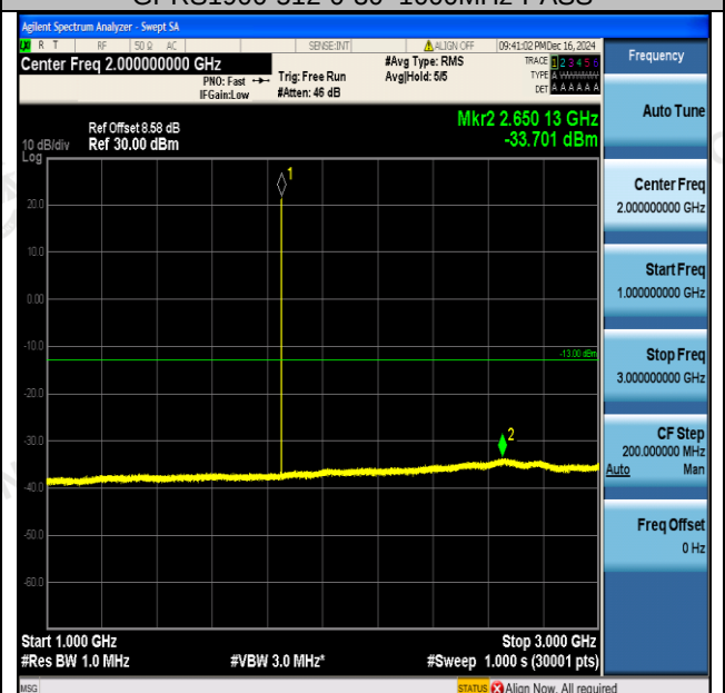
GPRS1900-512-0-1000-3000MHz-PASS
