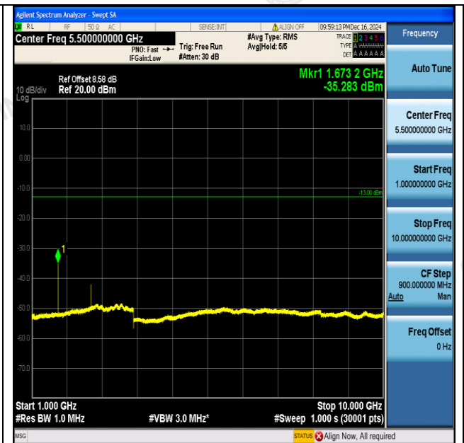
GPRS850-190-5-1000~10000MHz-PASS
