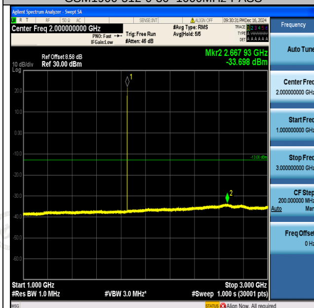
GSM1900-512-0-1000-3000MHz-PASS
