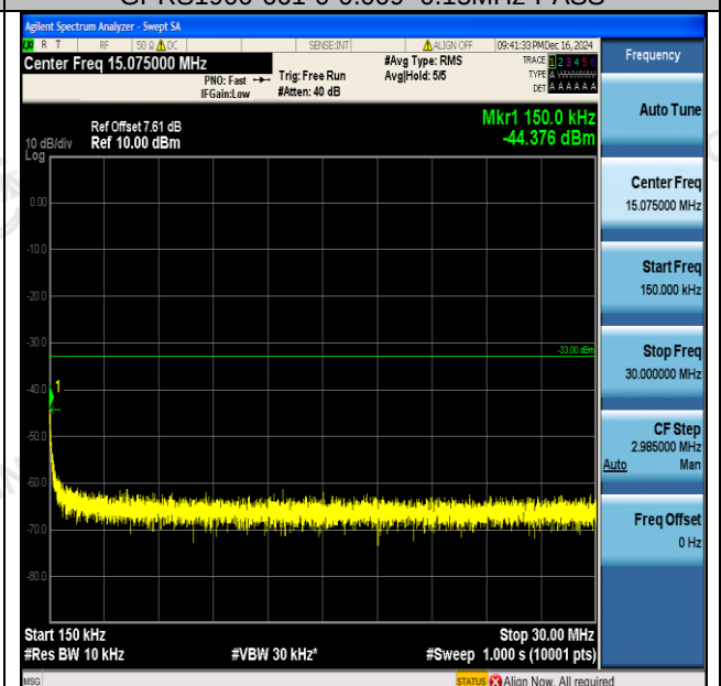
GPRS1900-661-0-0.15~30MHz-PASS
