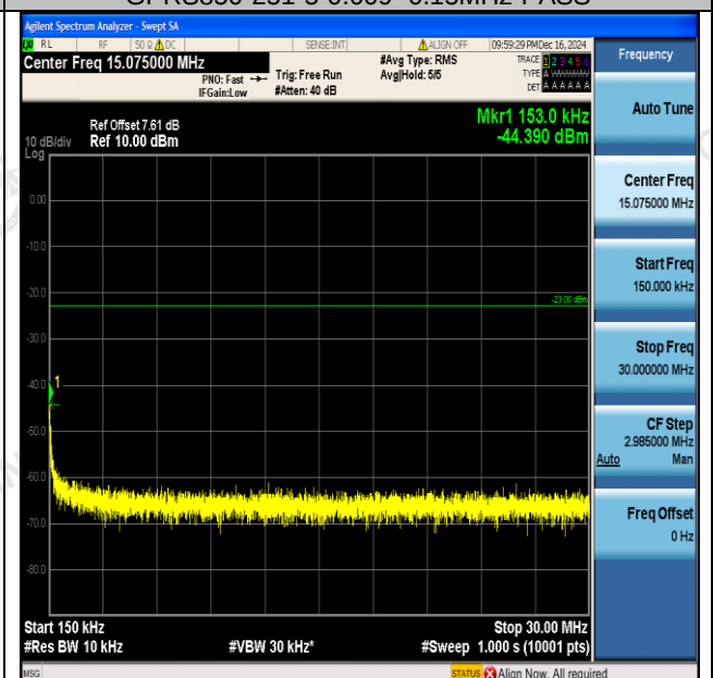
GPRS850-251-5-0.15~30MHz-PASS
