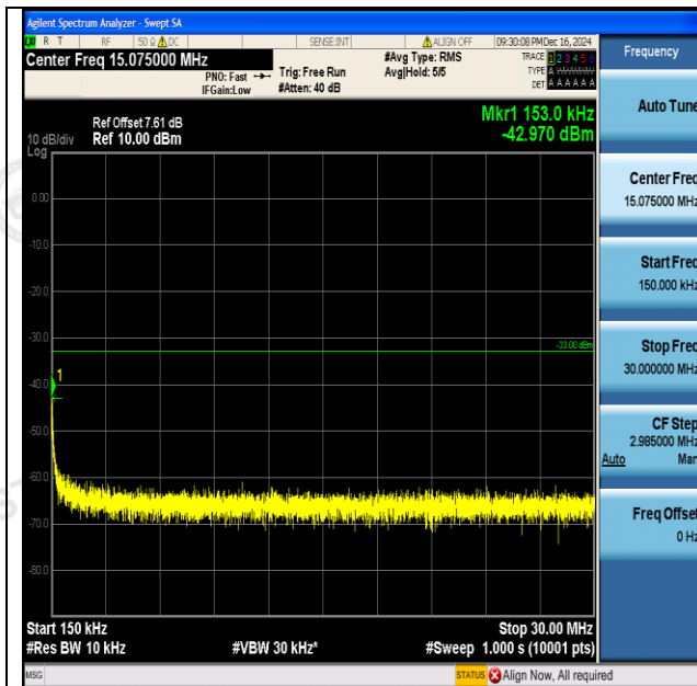
GSM1900-512-0-0.15-30MHz-PASS
