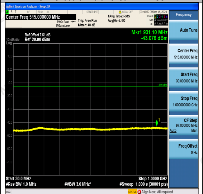
GPRS1900-512-0-30-1000MHz-PASS
