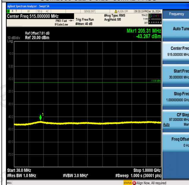
GSM1900-512-0-30-1000MHz-PASS
