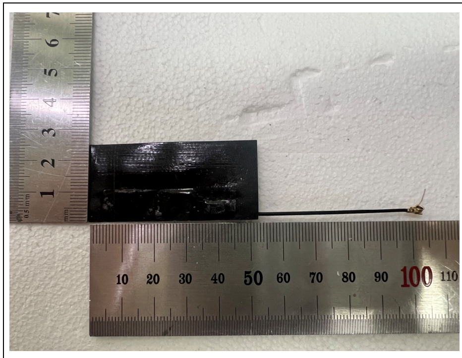
LTE Antenna
